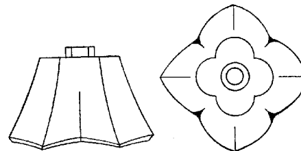
Turmhelm Für 4 Walm zu W 5 oder W 7 passend
