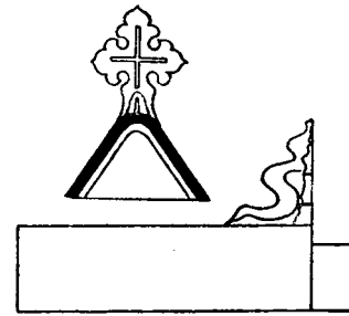
WV 9 + WV 10 Spitzer Walmziegel W 4 mit Krabben WV 9 = 35 cm WV 10 = 25 cm
