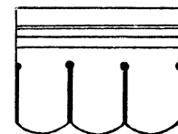
W 11 Kleiner Seitenziegel zu Z 2,3,+4 Länge= 25 cm Breite = 18 cm W 11 b Breite= 15 cm
