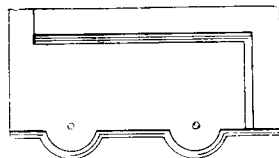
W 10 Seitenziegel zu Z 1 wird rechts und links gefertigt
