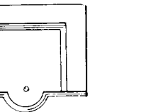
W 18 Seitenziegel zu Z 2+Z 16 Decklänge: 33 cm 1m Sparren = 3 Stück
